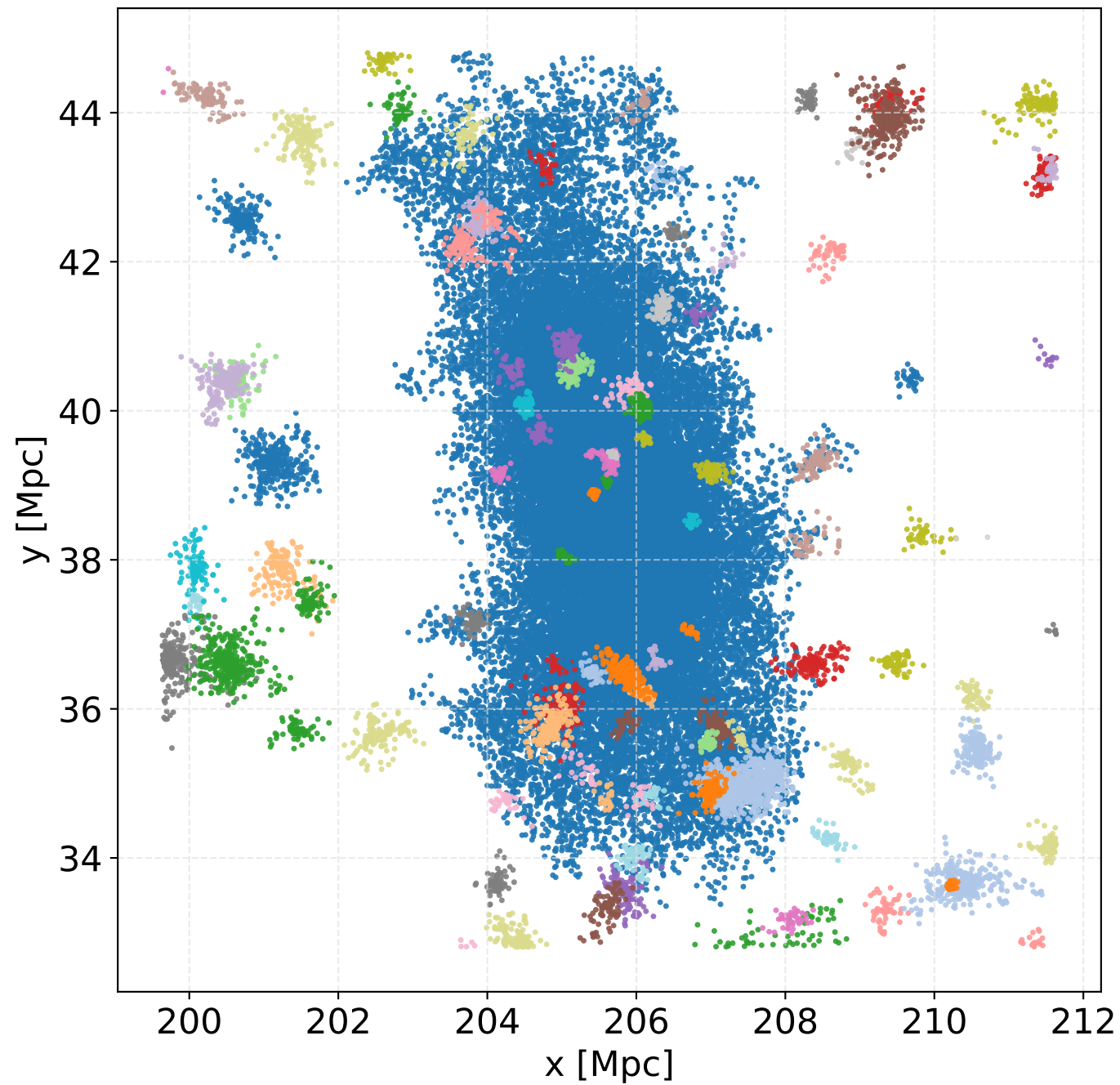
SUBFIND Particles
